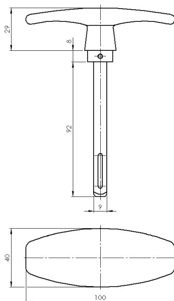
T-Griff
